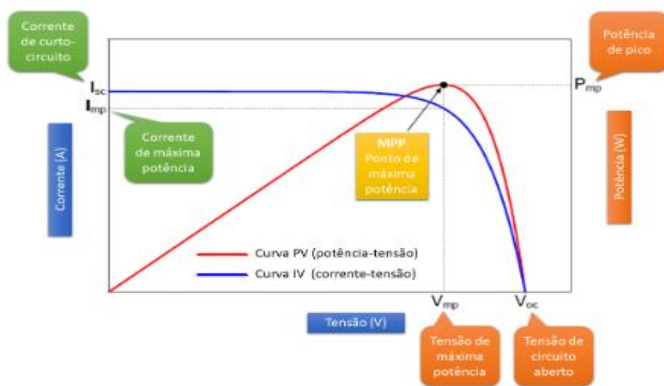
Figura 3- Explicação da curva de uma célula fotovoltaica
