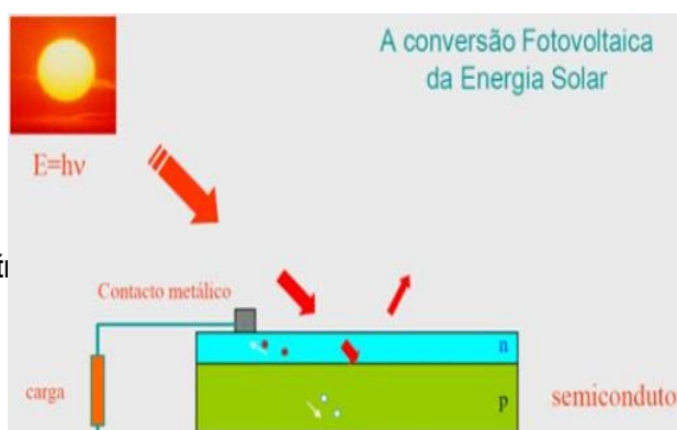
Figura 4- Efeito fotovoltaica
